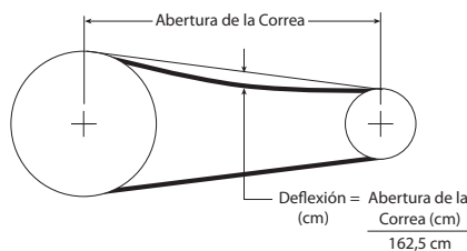
Figura 7 — Tensión de la Correa
