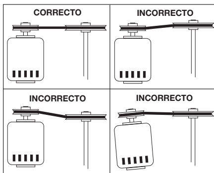
Figura 6 — Alineación de las Poleas
