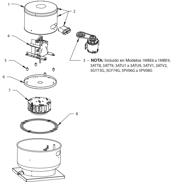
Figura 9 — Ilustración de Repuestos para Extractores Centrífugos de Transmisión por Correa de Tiro Hacia Arriba
